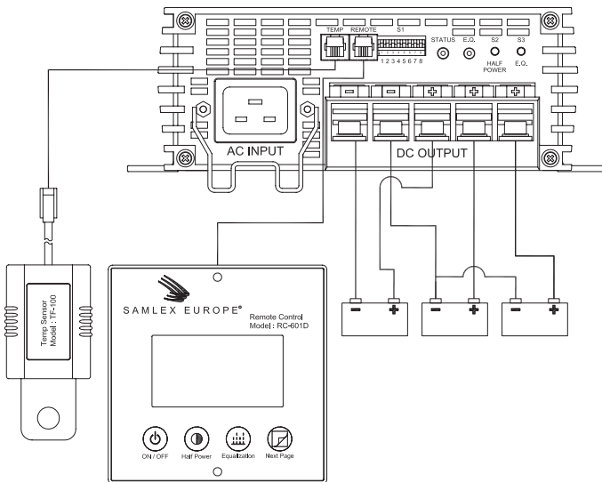
Afbeelding 5 Aansluiten
