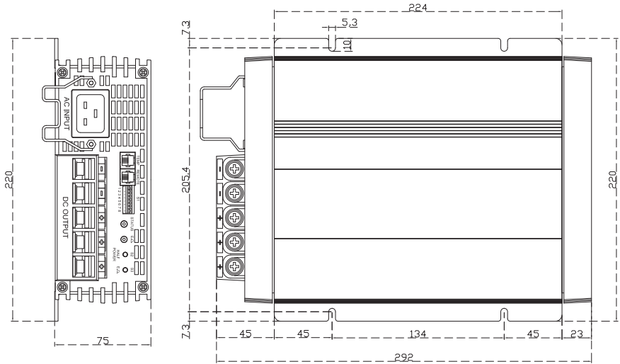
Afbeelding 3a WSC-1250Li / WSC-2425Li lader bovenaanzicht (mm)
