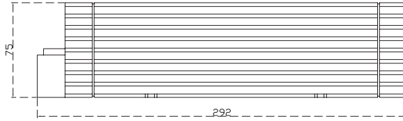
Afbeelding 4a WSC-1250Li / WSC-2425Li lader zijzichts (mm)
