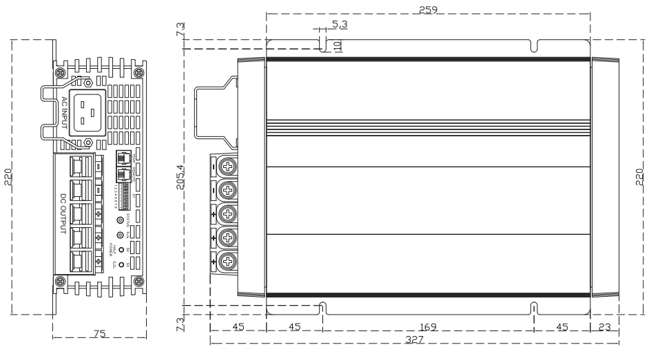
Afbeelding 3b WSC-1280Li / WSC-2440Li / WSC-4820Li lader bovenaanzicht (mm)
