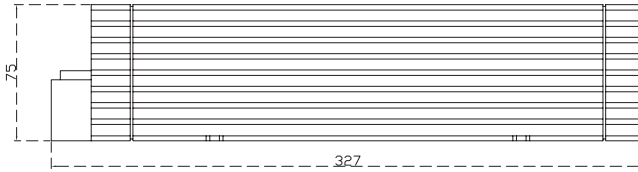
Afbeelding 4b WSC-1280Li / WSC-2440Li / WSC-4820Li lader zijzichts (mm)
