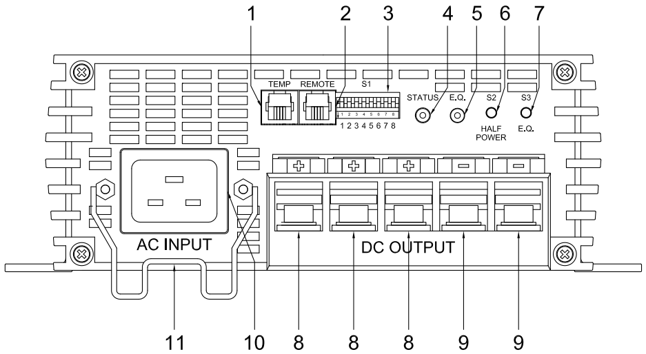
Figura 1 Vista frontal del cargador WSC-12120Li / WSC-2460Li / WSC-4830Li
