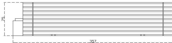
Figura 4 Vista lateral del cargador WSC-12120Li / WSC-2460Li / WSC-4830Li (mm)
