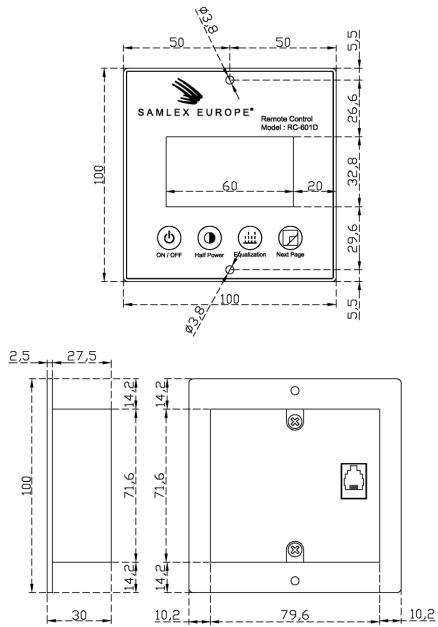
Figura 13 Dimensiones del control remoto RC-601D (mm)
