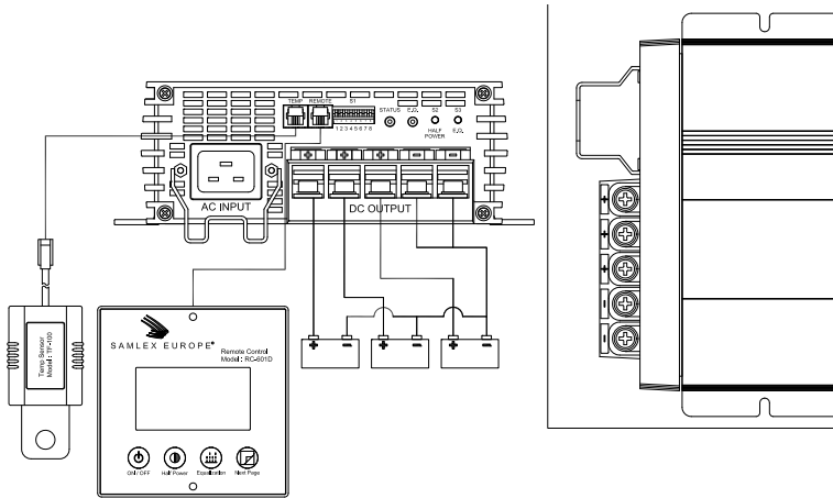
Figura 5 Haciendo conexión
