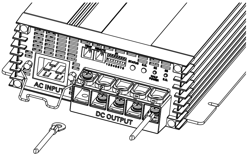
Figura 6 Configuración de los cables
